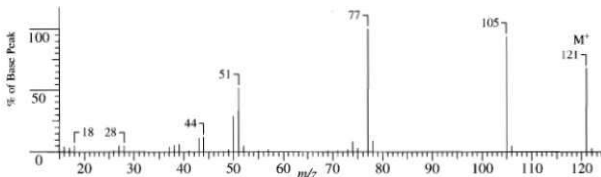
Figure IV.6 Spectre de masse IE de la benzamide.
