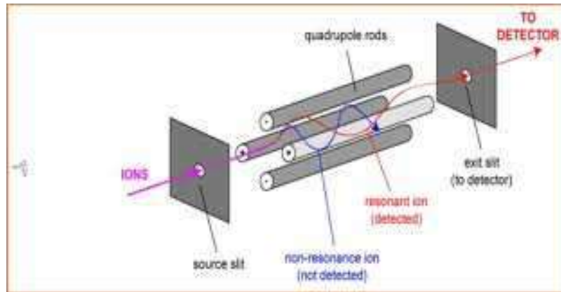
Figure IV.9 Schéma d'un spectromètre de masse à quadripôle.
