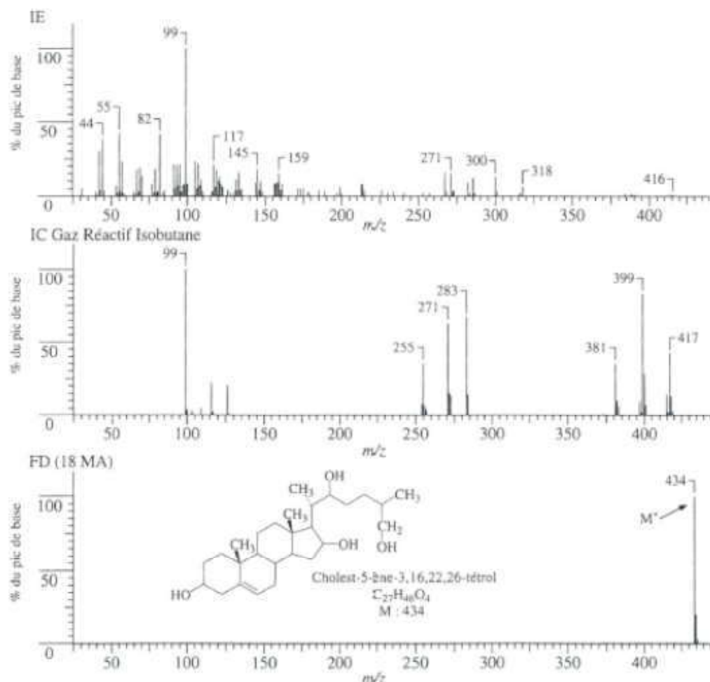
Figure VI.2 : Spectre de masse IE, IC et FD du cholest-5-ène-3,16,22,26-tétrol.
